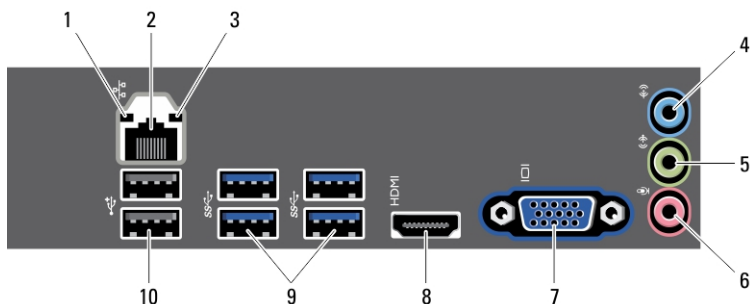
图 2: 背面板视图
